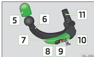
Obr. 118 Tažné rameno
