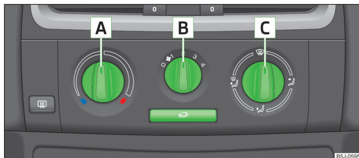
Obr. 95 Topení: ovládací prvky
