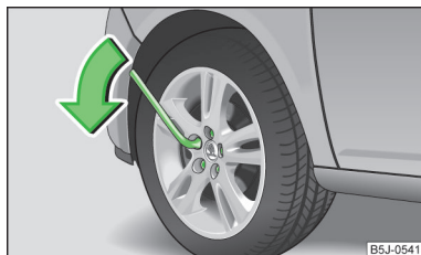
Obr. 141 Výměna kola: povolení šroubů
