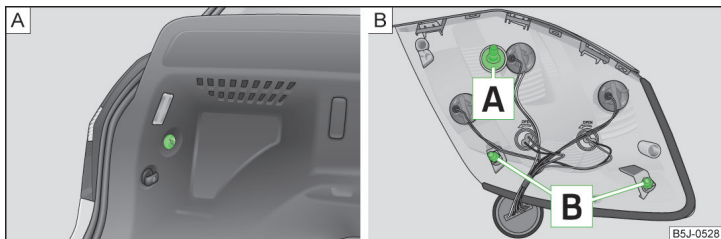
Obr. 162 Plastová matice / zadní skupinová svítidla
