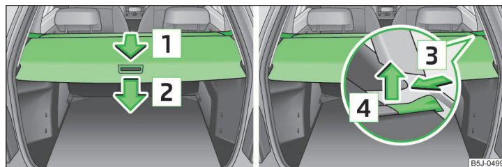
Obr. 66 Zavazadlový prostor: roletový kryt / demontáž roletového krytu
